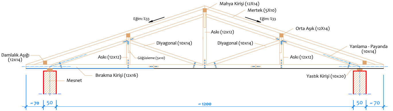
ÜÇ ASKILI AHŞAP ASMA ÇATI MAKASI
