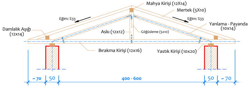
TEK ASKILI AHŞAP ASMA ÇATI MAKASI
