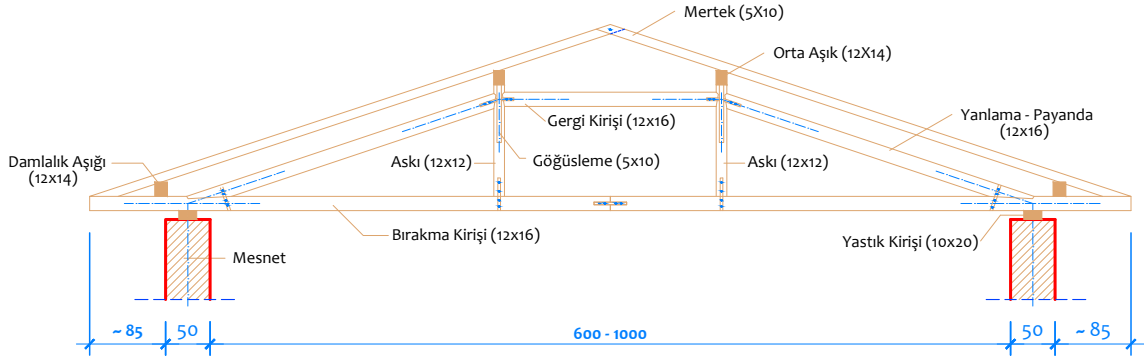
İKİ ASKILI AHŞAP ASMA ÇATI MAKASI
