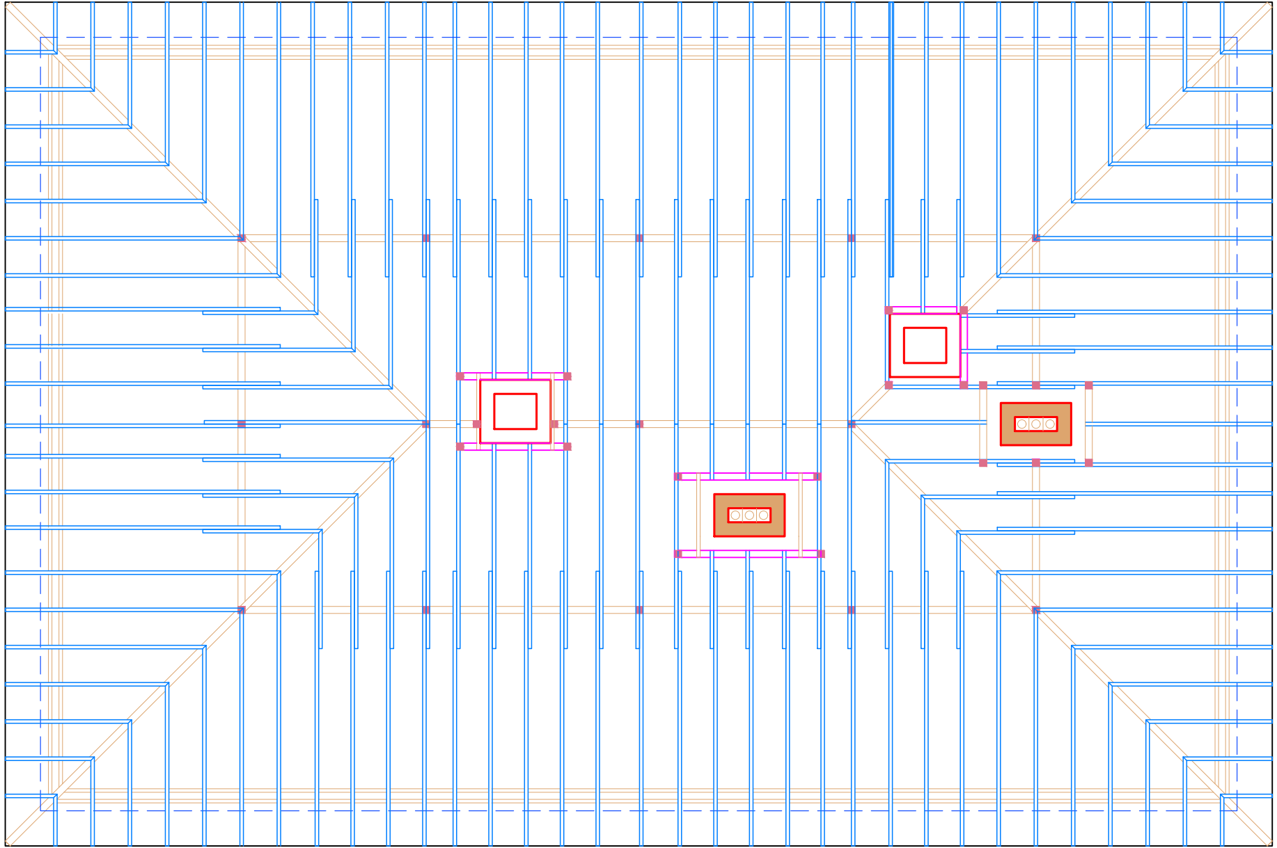
AHŞAP OTURTMA ÇATIDA BACA KASNAKLAMALARI
