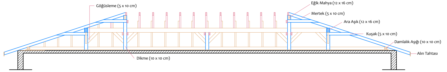
Boy Kesit
