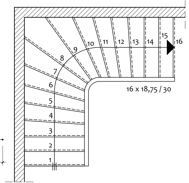
DENGELENDİRİLMİŐ MERDİVEN PLANI
