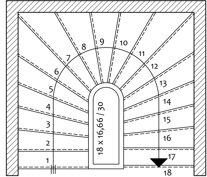
DENGELENDİRİLMİŐ MERDİVEN PLANI
