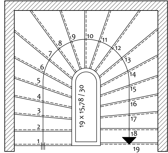
DENGELENDİRİLMİŞ MERDİVEN PLANI
