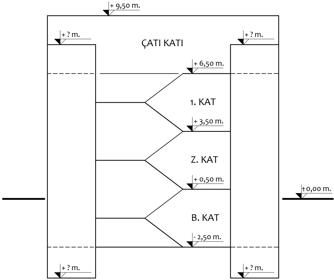
ŞEMATİK KESİT
