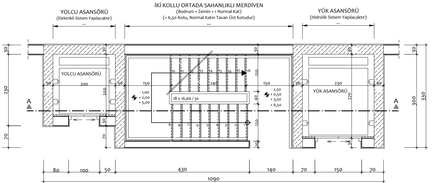
ZEMİN KAT ÇEKİRDEK PLANI ÖLÇEK: 1/50
