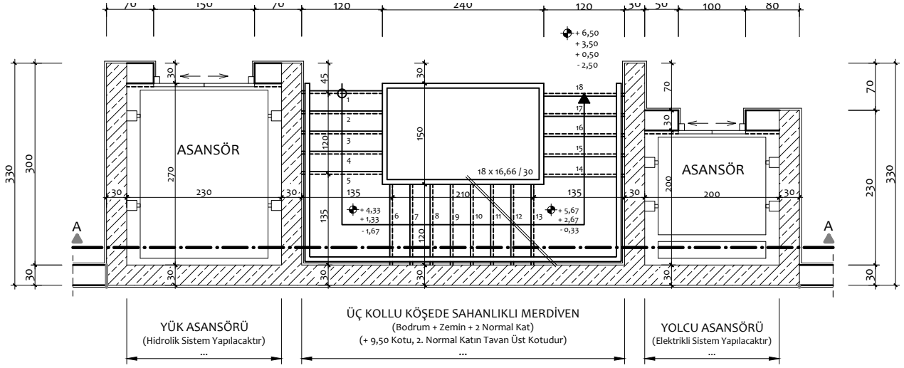
ÇEKİRDEK PLANI / ÖLÇEK: 1/50
