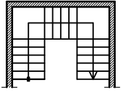
ÜÇ KOLLU KÖŞEDE SAHANLIKLI MERDİVEN
