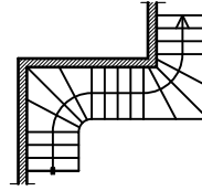
ÜÇ KOLLU ÇEYREK TERS DÖNER MERDİVEN
